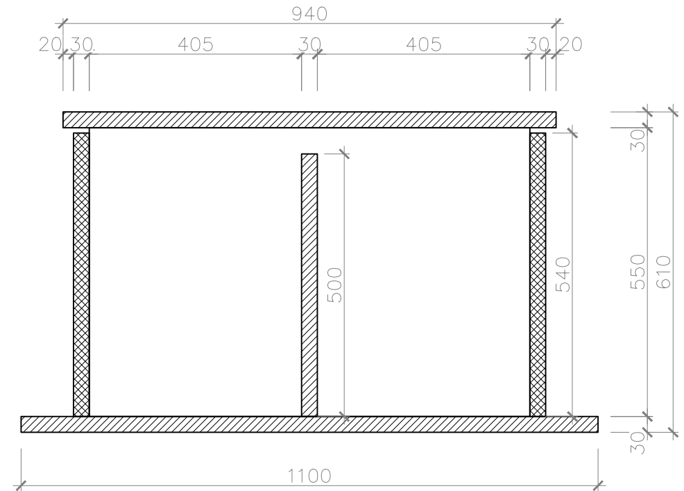
SVISLÝ ŘEZ B
