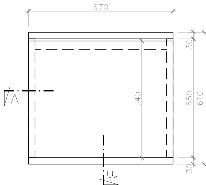
POHLED ČELNÍ
