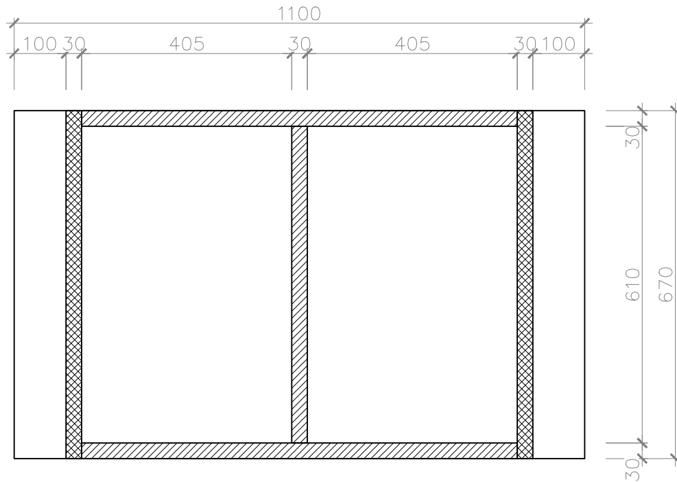
PŮDORYSNÝ ŘEZ A
