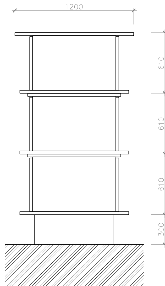
POHLED BOČNÍ
