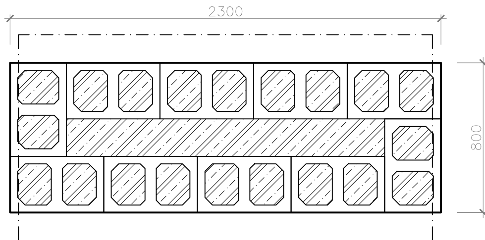
PŮDORYS ZÁKLADŮ
