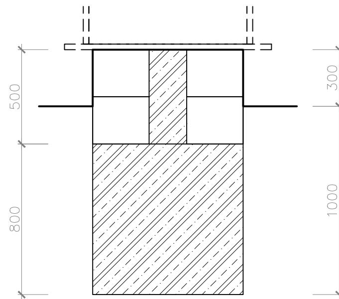
PŘÍČNÝ ŘEZ
