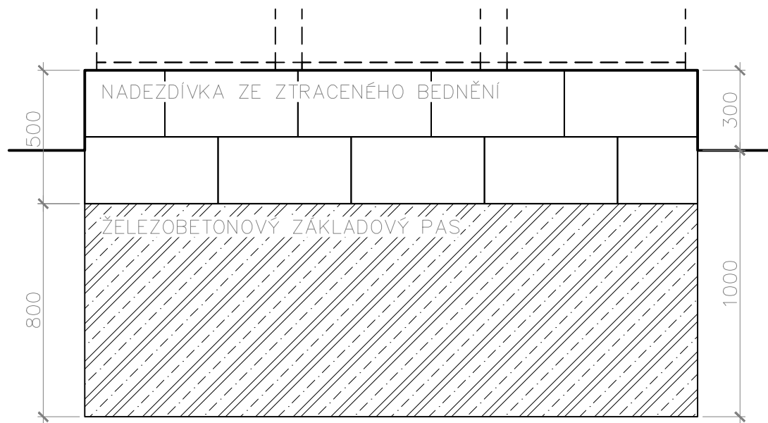
PODÉLNÝ ŘEZ
